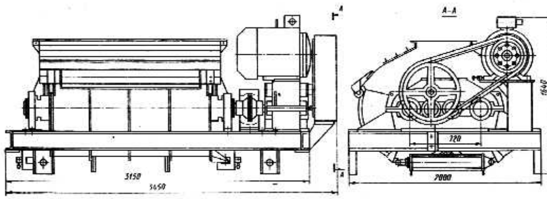
ნახ. 12.4. ღარული ორლილვა ბეტონსარევი
