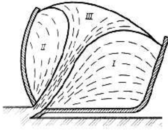
ნახ. 8.4. სკრეპერის ციცხვის შევსების სქემა
