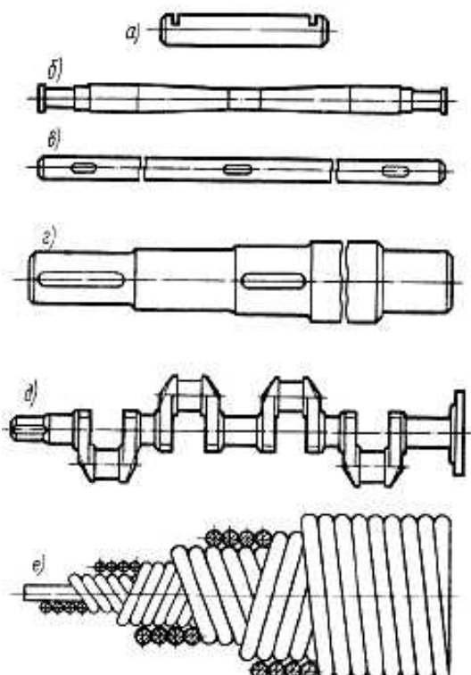
ნახ. 5.11. ლილვებისა და ლერძების ძირითადი სახეები
