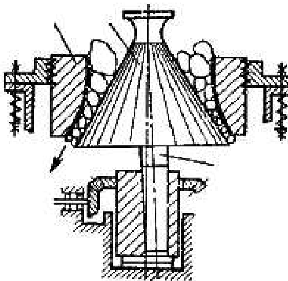
ნახ. 9.5. კონუსური სამსხვრეველი:
