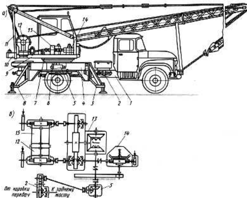
ნახ. 10.7. საავტომობილო ამწე
