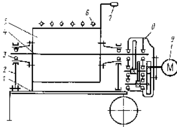
ნახ. 12.6. ხსნარის მოსამზადებელი პერიოდული ქმედების შემრევი (ჰორიზონტალური ლილვით):
