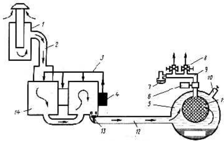
ნახ. 5.2. კომპრესორული დანადგარის (სადგურის) საერთო სქემა
