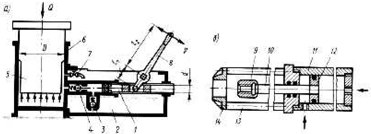
ნახ. 10.3. ჰიდრავლიკული დომკრატი: ა - ხელის ამძრავით; ბ - ღერძის გასაჭიმში მოწყობილობა
