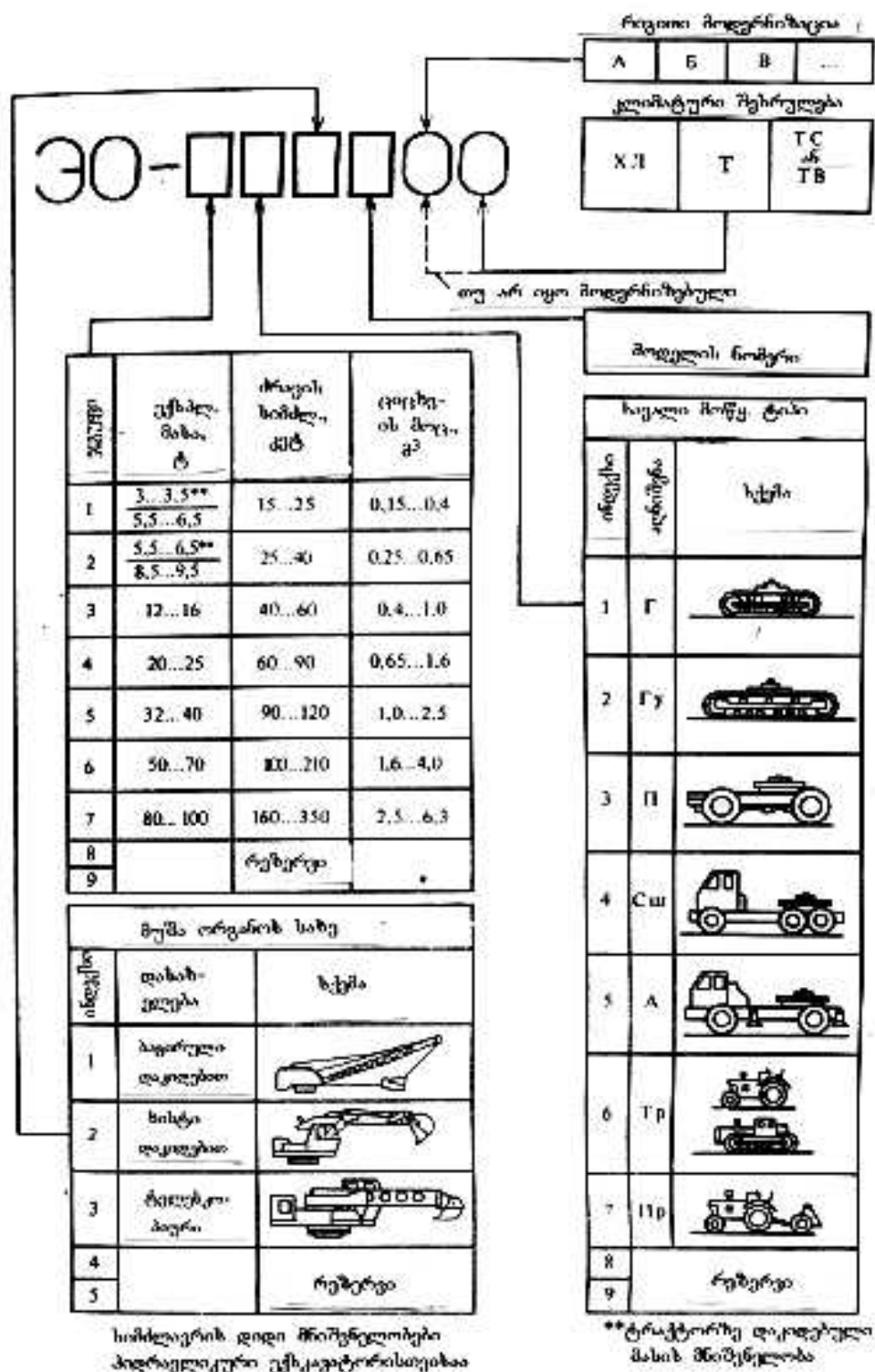
ნახ. 13.1 ერთიცხვანი სამშენებლო უწყკავატორების ინდექსების სტრუქტურა
